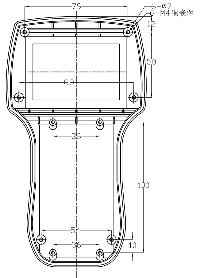
上盖底视图
